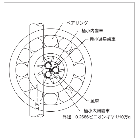
ピニオン歯車を組み込んだ 超小型遊星歯車回転機構の概念図
